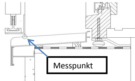
T-Profil mit Winkel über der FB
