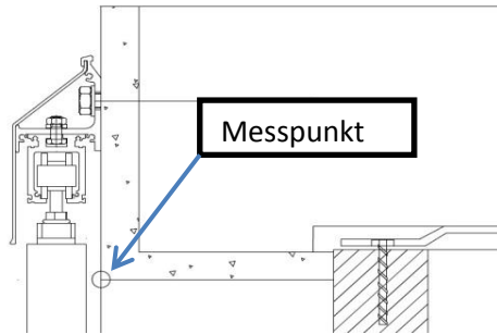
Trägerprofilset
