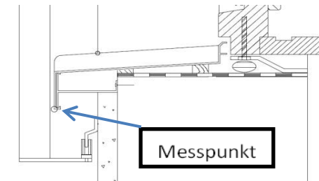
Z-Profil unter der Fensterbank
