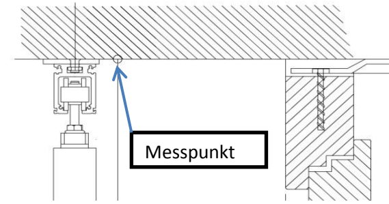
Deckenmontageset Comfort
