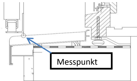
Punktführung
